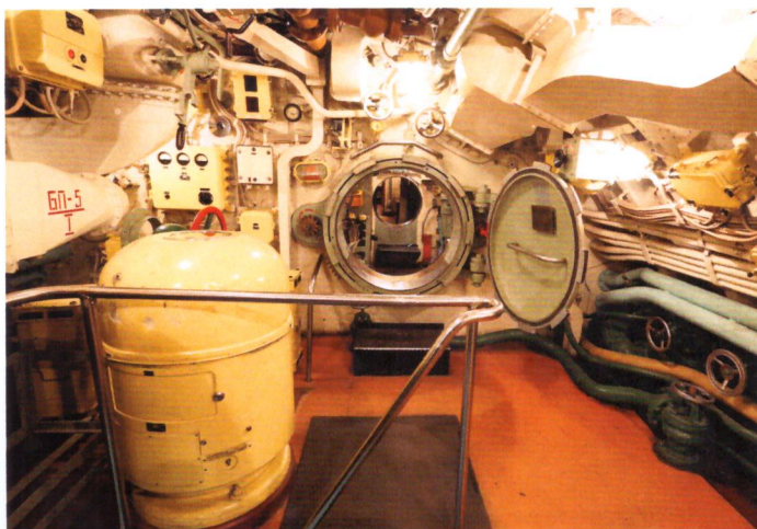
Гирокомпас (на переднем плане слева) в отсеке № 5
