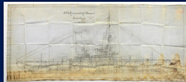
Чертеж линейного корабля «Байерн» (S.M. Linien Schiff «Bayern»). Продольный разрез. Масштаб 1 : 100 Германия, 1913-1916
